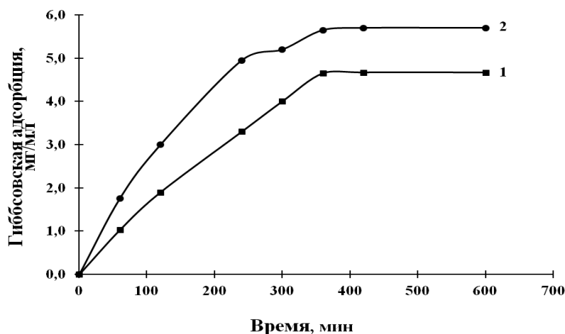
Рис. 3. Влияние молекулярной массы аппрета на Гиббсовскую адсорбцию: 1 – 1-ПГЭф, 2 – 2-ПГЭф
