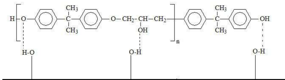
Рис. 5. Образование водородных связей между стекловолном и ПГЭф
