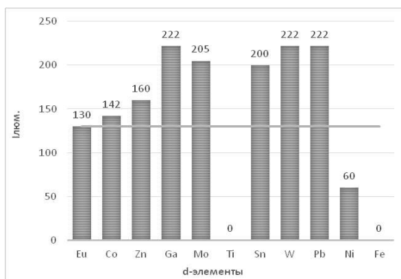
Рис. 7. Влияние d-элементов на I_{\text{люм}} раствора комплекса Еу с Нол в мицеллярной среде: C_{\text{Еу}} = C_{\text{d-эл}} = C_{\text{ДЦПХ}} = C_{\text{Нол}} = 1 \cdot 10^{-3} \text{М} ; V_{\text{Еу}} = V_{\text{d-эл}} = V_{\text{ДЦПХ}} = 1 \text{ мл} ; V_{\text{Нол}} = 3 \text{ мл} ; \lambda = 614 \text{ нм} ; рН = 8,0; V = 10 \text{ мл} ; l = 1 \text{ см}
