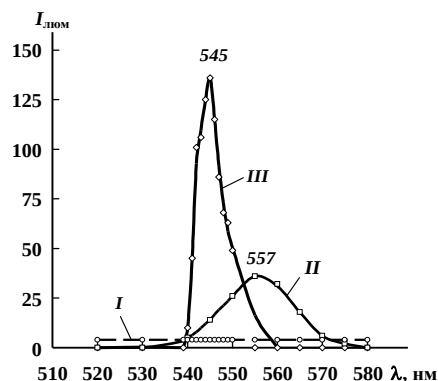
Рис. 3. Зависимости I_{\text{люм}} от длины волны для растворов Tb (I), нолицина (II) и комплекса Tb с НОЛ (III), C_{\text{Tb}} = C_{\text{НОЛ}} = 1 \text{ мл } 1 \times 10^{-3} \text{ М} ; \text{pH} = 6,0 ; V = 10 \text{ мл} ; l = 1 \text{ см}
