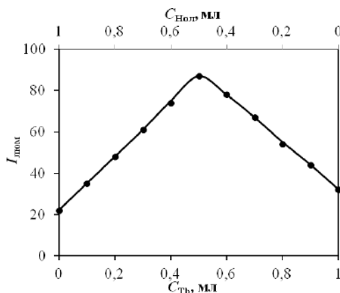
Рис. 4. Определение состава комплекса Tb с НОЛ методом изомолярных серий. C_{\text{Tb}} = C_{\text{НОЛ}} = 1 \times 10^{-3} \text{ М} , \lambda = 545 \text{ нм} , \text{pH} = 5,9 , V = 10 \text{ мл} , l = 1 \text{ см}
