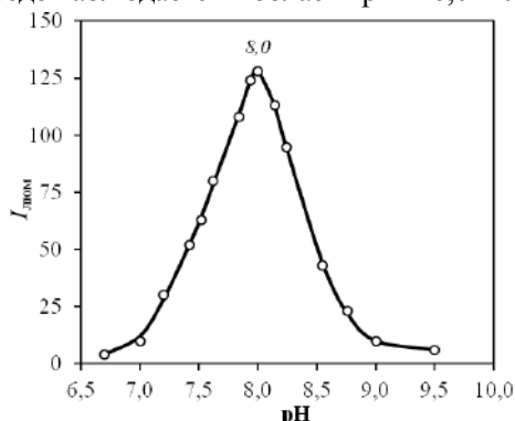
Рис. 5. Зависимость I_{\text{люм}} раствора комплекса Еу с Нол в мицеллярной среде от рН среды: C_{\text{Еу}} = C_{\text{ДЦПХ}} = C_{\text{Нол}} = 1 \cdot 10^{-3} \text{М} ; V_{\text{Еу}} = V_{\text{ДЦПХ}} = 1 \text{ мл} ; V_{\text{Нол}} = 1,5 \text{ мл} ; \lambda = 614 \text{ нм} ; V = 10 \text{ мл} ; l = 1 \text{ см}
