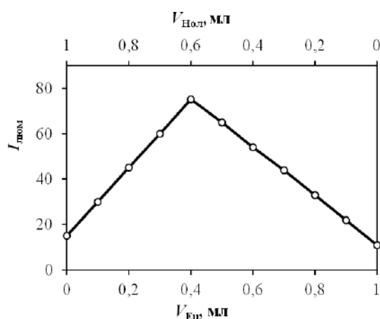
Рис. 3. Определение состава комплекса Eu с Нол методом молярных отношений: C_{Eu} = C_{Нол} = 1 \cdot 10^{-3} \text{ М} ; C_{ДЦПХ} = 1 \text{ мл } 1 \cdot 10^{-3} \text{ М} ; \lambda = 614 \text{ нм} ; \text{pH} = 8,0 ; V = 10 \text{ мл} ; l = 1 \text{ см}
