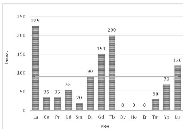
Рис. 6. Влияние других РЗЭ на I_{\text{люм}} раствора комплекса Еу с Нол в мицеллярной среде: C_{\text{Еу}} = C_{\text{Нол}} = C_{\text{ДЦПХ}} = 1 \cdot 10^{-3} \text{М} ; V_{\text{Еу}} = V_{\text{ДЦПХ}} = V_{\text{РЗЭ}} = 1 \text{ мл} ; V_{\text{Нол}} = 3 \text{ мл} ; \lambda = 614 \text{ нм} ; рН = 8,0; V = 10 \text{ мл} ; l = 1 \text{ см}
