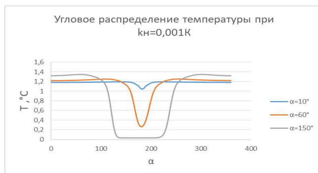
Рис. 2. Угловое распределение температуры при k_n=0,001 К при углах распределения неоднородности 10, 60, 150°
