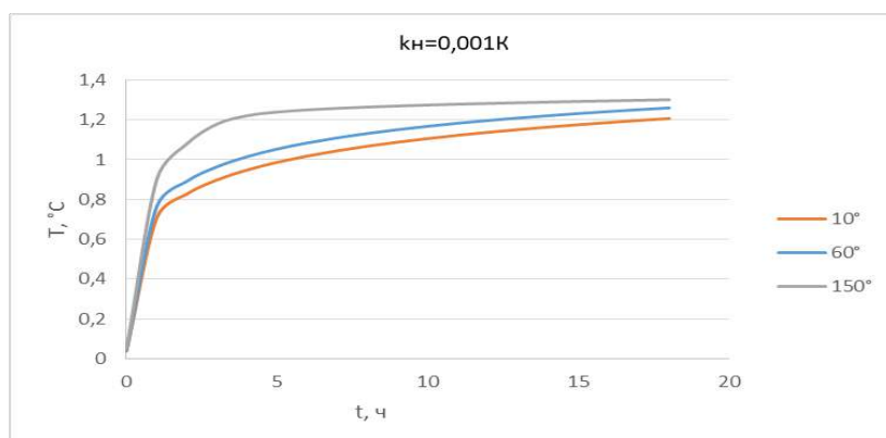
Рис. 1. График зависимости изменения температуры от времени при различных углах распределения неоднородности (10, 60, 150°) при k_n=0,001 К
